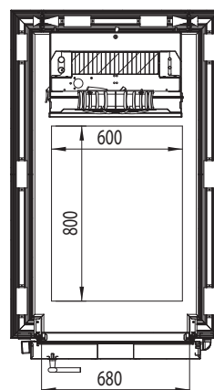
SEZIONE A-A
